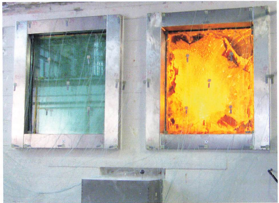
Einzigartig: Walter Wurster hat als erster Hersteller weltweit eine Festverglasung in F120 im Sortiment
