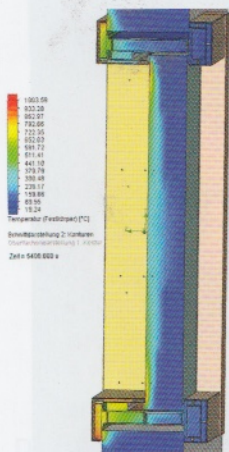
Das Simulationsprogramm zeigt kritische Wärmeübergänge auf und wie die Hitze 'kriecht'. Blauer Bereich: Verzögerte Wärmeausbreitung.
