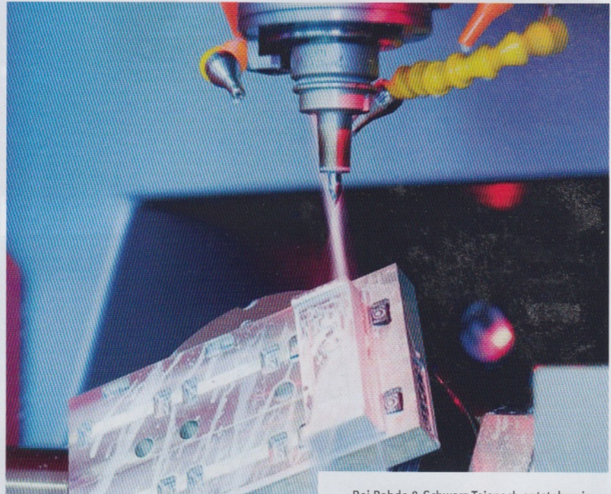
Bei Rohde & Schwarz Teisnach entstehen in großer Fertigungstiefe Gehäuse, Außenkörper, Wellen oder Rahmen und Anschlussstücke für die anspruchsvollen Produkte. ©Rohde & Schwarz
