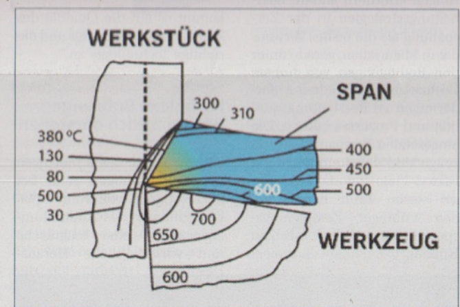
Messungen bescheinigen den Arno ACS-Werkzeugen mit Innenkühlung eine Reduzierung der Temperatur auf etwa die Hälfte
