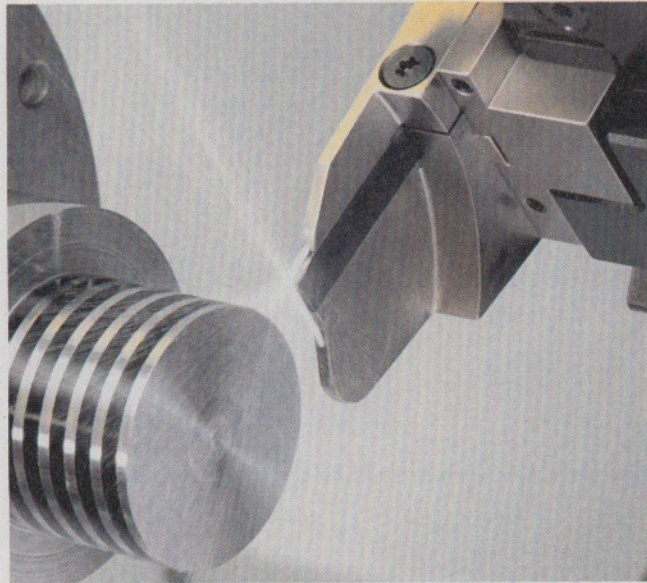
Mit Innenkühlung durch clevere und hochfeine Kanalführungen gelingt es Werkzeugherstellern wie Arno Werkzeuge, den Kühlschmierstoff direkt in die Schneid- und damit in die Problemzone zu führen
