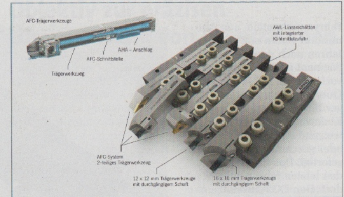
Auch beim Langdrehen mit häufig zu wechselnden Werkzeugen, müssen Anwender nicht auf integrierte Kühlung verzichten: Arno AWL und AFC ist ein Werkzeugschnellwechselsystem mit innerer Kühlung
