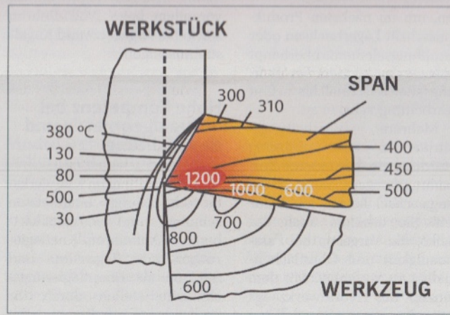
Messungen bescheinigen den Arno ACS-Werkzeugen mit Innenkühlung eine Reduzierung der Temperatur auf etwa die Hälfte
