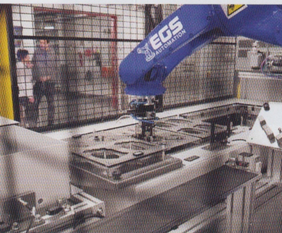
Hat der Knickarmroboter ein Rohteil entnommen, positioniert er es passgenau in der Vorrichtung.
