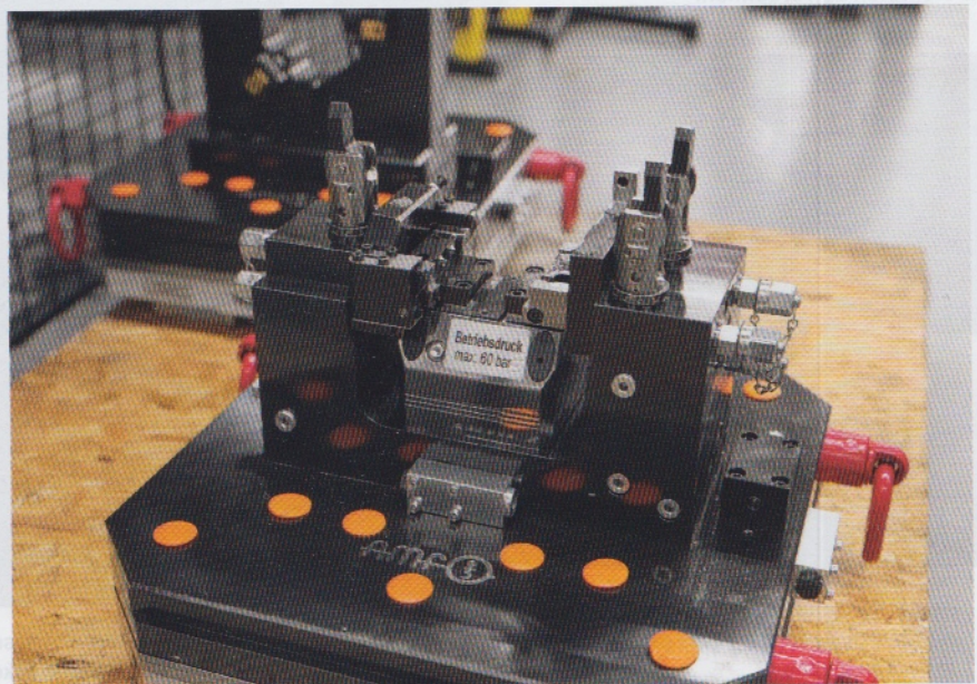
Gespannt werden die Rohteile in der AMF-Vorrichtung hydraulisch mit maximal 190 bar Druck.
