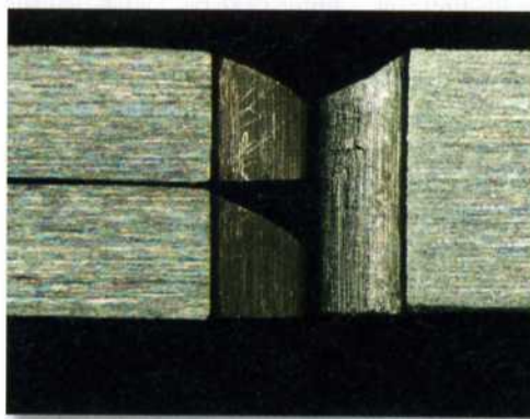
Zahnrad mit reduziertem Stanzeinzug. Bild: Fritz Schiess AG
