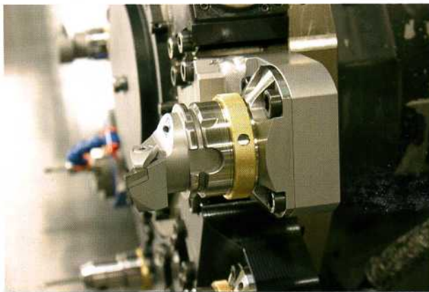
Bild 2: Die Bär + Mettler AG hat für das Hartdrehen zusammen mit der Swiss Tool Systems AG den Revolver auf einer Hardinge-Drehmaschine mit HSK-T ausgestattet und erzielt damit sensationelle Ergebnisse
