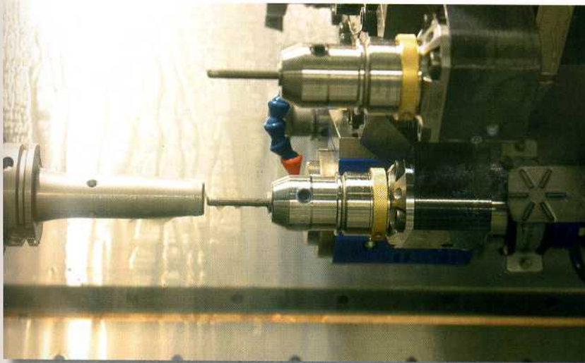
Bild 4: „Vor allem beim Bohrungsdrehen von kleinen Durchmessern in gehärteten Werkstücken ist die hohe Stabilität der Swiss-Flex HSK-Schnittstelle auf der Hardinge Maschine optimal“
