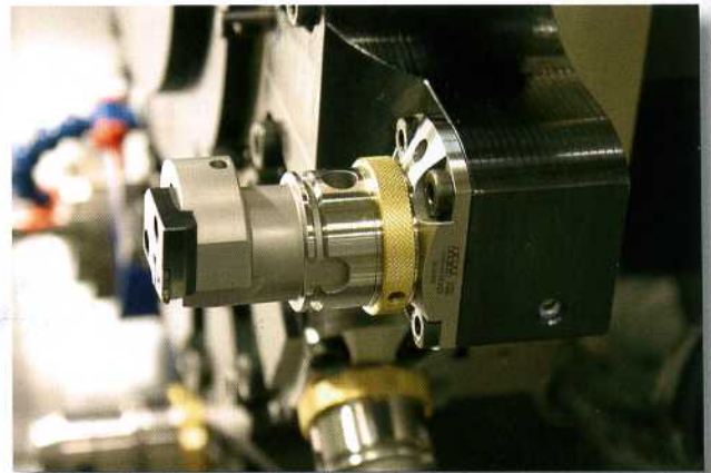
Bild 3: HSK-T ermöglicht schnelle Werkzeugwechsel. Was früher mehr als zehn Minuten dauerte, ist heute in zwei Minuten erledigt
