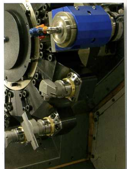
Bild 6: Auch angetriebene Werkzeuge können auf der HSK-Schnittstelle der Drehmaschine eingesetzt werden. Genauigkeiten mit Toleranzen bis 1 µm werden realisiert (Werkbilder: Bär + Mettler AG, Swiss Tool Systems AG, Hardinge GmbH, CH-Bürglen)
