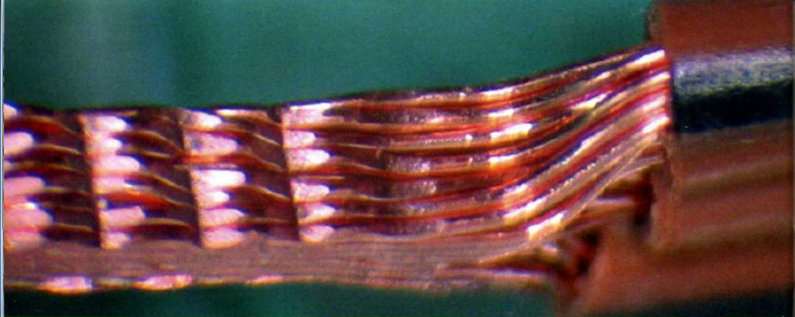
Sichere Ultraschall-Schweißverbindung aller Drähte mehrerer Litzen. Bilder: Telsonic
