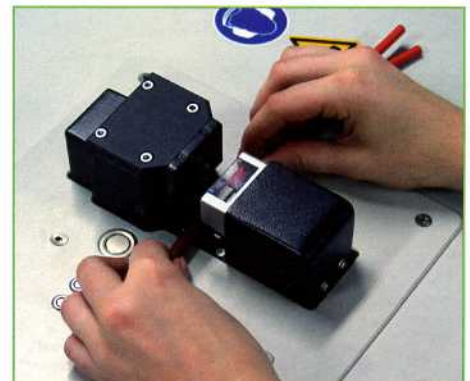
Ein Einlegeraum von 10 x 19 mm ermöglicht das Verschweißen von Litzenknoten großer Querschnitte bis 45 mm 2
