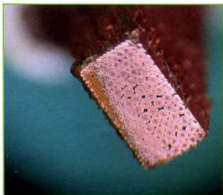
Zur Kontrolle aufgesägter Querschnitt und Schliffbild einer Ultraschall-Schweißverbindung
