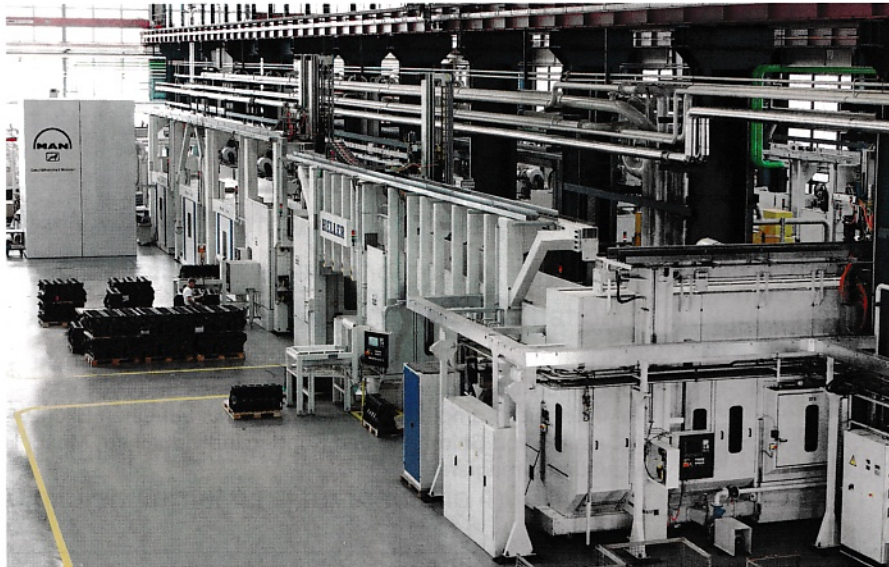
Bild 4: Stark in der Automobilindustrie: komplettes Fertigungssystem von Heller für die Kurbelgehäusefertigung beim Nutzfahrzeughersteller MAN
