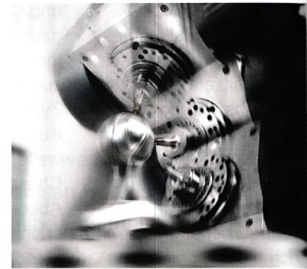
Bild 5: Wichtiger Partner für die Erstausrüstung: Heller ist einer der führenden Anbieter von fünfachsigen Bearbeitungszentren für Fräs- und Fräsdreh-Prozesse
