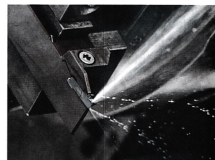
Bild 12: Kühlung direkt in der Schnittzone: die innengekühlte zweischneidige Wendeschneidplatte Typ S224 von Paul Horn
