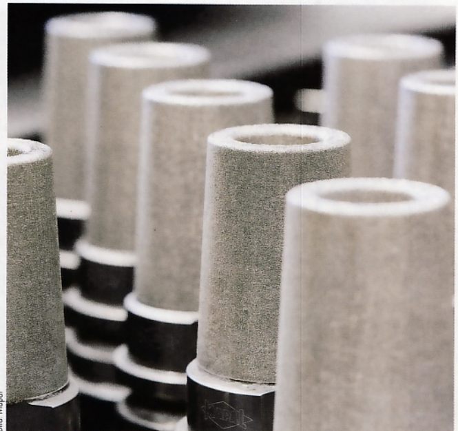
Teilweise additiv gefertigtes Hydrodehnspannfutter von Mapal: Ohne Lötstelle ist es deutlich temperaturbeständiger als sein konventionelles Pendant.
