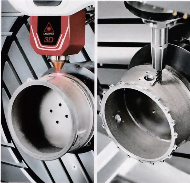
Technologieintegration von DMG Mori: Laserauftragschweißen und 5-Achs-Fräsen intelligent kombiniert.
