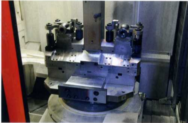
Bild 5: Die Experten von Röhm haben eine drehbare und hydraulisch betätigte 2-fach-Spannvorrichtung gebaut
