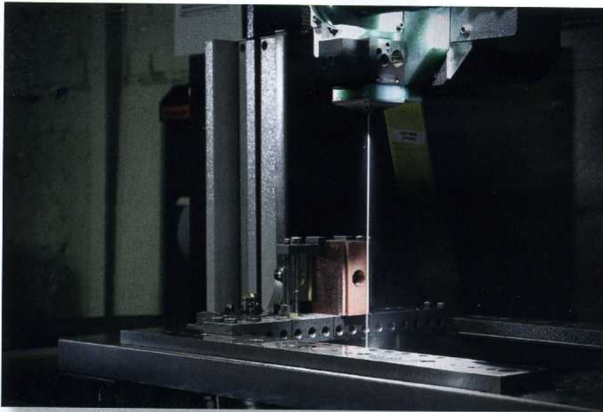
Bild 4: Ein einziges Drahtführungssystem der CUT 2000 ermöglicht die Benutzung von verschiedenen Drahtdurchmessern. Dabei wird der Draht zuverlässig automatisch eingefädelt, indem er offen in einem Wasserstrahl geführt wird
